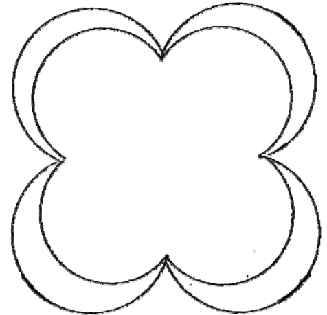
Lunel
